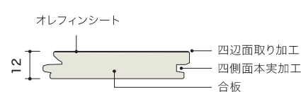
断面図
